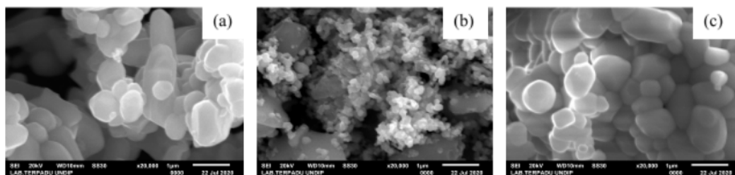
Gambar 2. Hasil SEM (a) \text{WO}_3 murni perbesaran 20.000 kali, (b) ZnO murni perbesaran 20.000 kali (c) Komposit \text{WO}_3\text{-ZnO} perbesaran 20.000 kali
