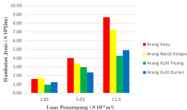
Gambar 2. Grafik Pengaruh Luas Penampang Terhadap Nilai Hambatan Jenis Resistor Arang Untuk Panjang Sedotan 0,02 m
