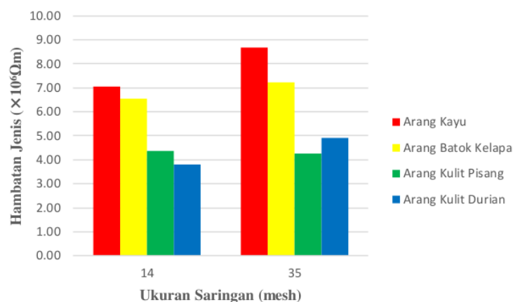
Gambar 3. Grafik Pengaruh Partikel Karbon Terhadap Nilai Hambatan Jenis
