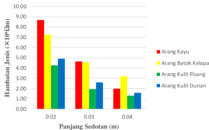
Gambar 1. Grafik Pengaruh Panjang Sedotan Terhadap Nilai Hambatan Jenis Resistor Arang Untuk Sedotan Besar
