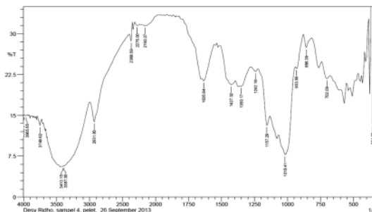
Gambar 3. Spektrum kulit singkong sebelum perlakuan.
