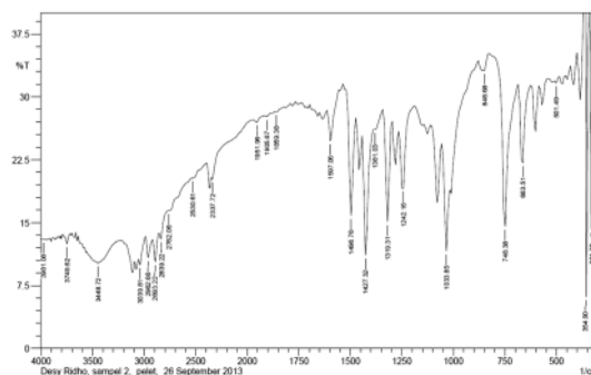
Gambar 5. Spektrum FTIR selulosa-MBT.
