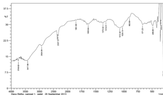
Gambar 4. Spektrum FTIR selulosa kulit singkong.
