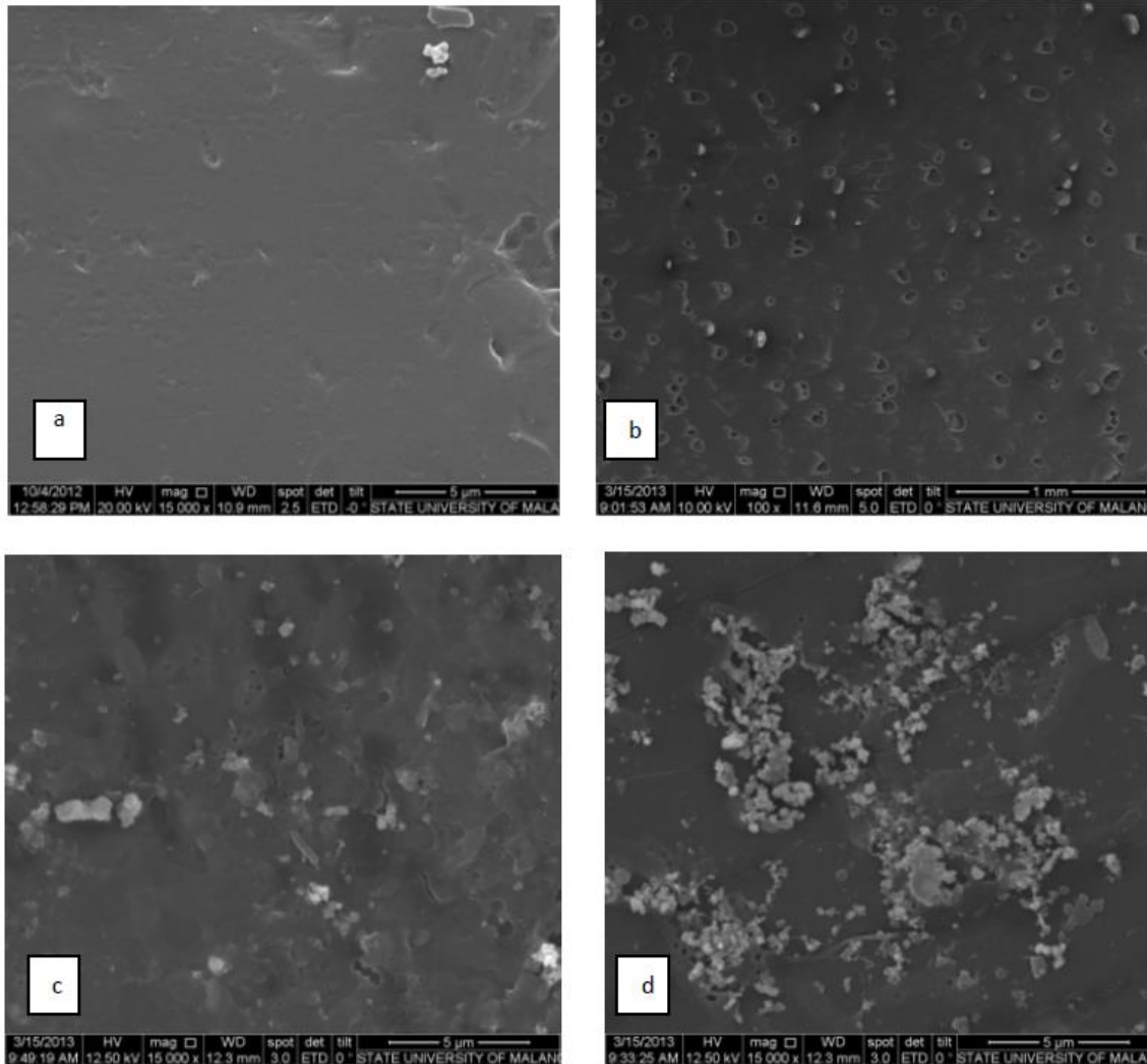
. Hasil SEM membran (a) membran baru (b) membran fouling emulsi bensin (c) membran fouling emulsi pelumas (d) membran fouling emulsi solar.
