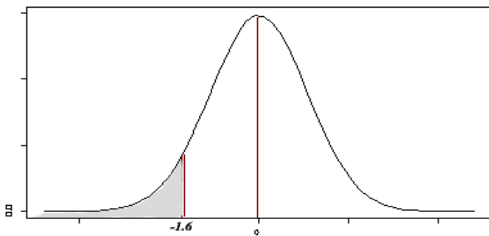
Gambar 3.8 P(Z < -1.6)
