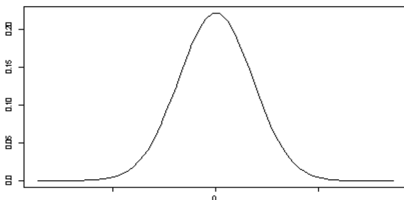
Gambar 3.1 Kurva Sebaran Normal
