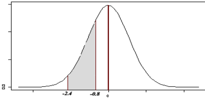
Gambar 3.7 P(-2.4 < Z < -0.8)
