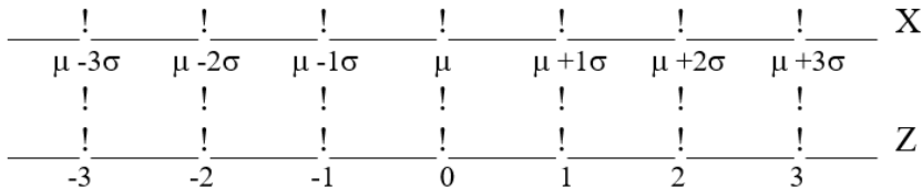
Gambar 3.4 Nilai variabel acak normal X dan Hasil Transformasi ke Normal Baku Z
