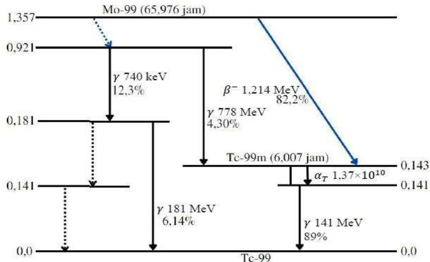
Gambar 2. Peluruhan Teknesium-99m (Tc-99m) (IAEA, 2007).
