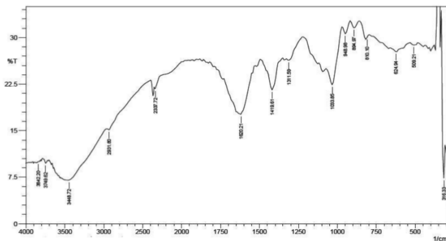
Gambar 2. Spektrum FT-IR Natrium Alginat
