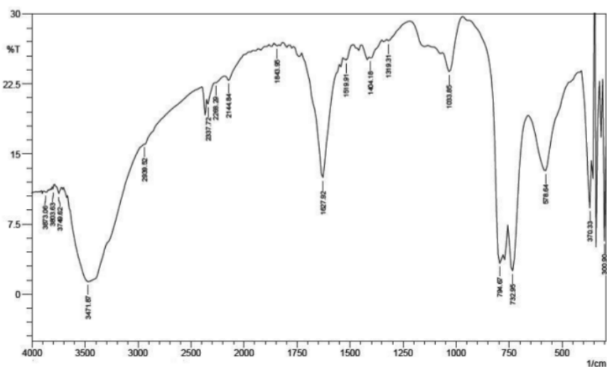
Gambar 4. Spektrum FT-IR Natrium Alginat Teroksidasi (Dialdehid Alginat)
