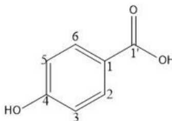
Gambar 1. Struktur senyawa 1
