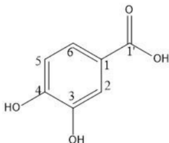
Gambar 2. Struktur senyawa 2
