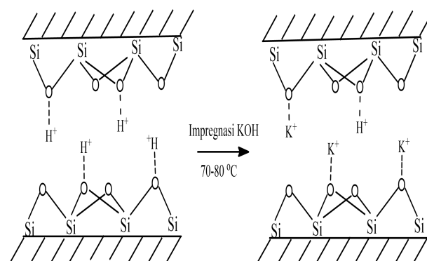
Gambar 2. Mekanisme impregnasi KOH pada DSBE
