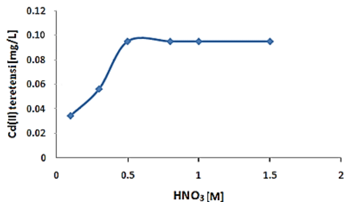
Gambar 5. Optimasi konsentrasi eluen \text{HNO}_3 .
