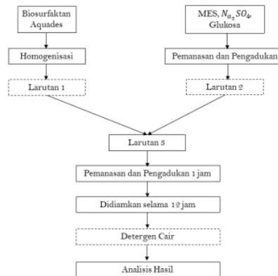
Gambar 2. Diagram Alir Pembuatan Detergen Cair
