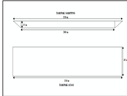
Gambar 3. Desain sumuran
