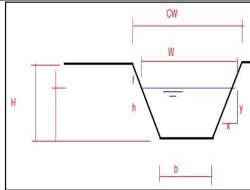
Gambar 4. Desain saluran terbuka trapesium
