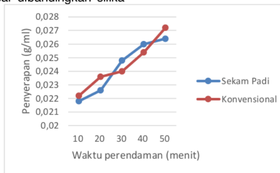
Gambar 2 Grafik Daya Serap Silika Gel Sekam Padi dan Silika Gel Konvensional
