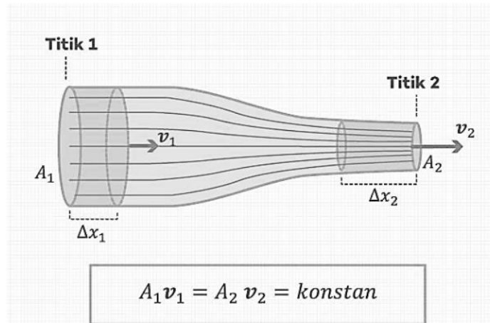
Gambar 1. Selang Pipa dengan Perbedaan Luas Penampang pada Persamaan Kontinuitas (Sumber: https://www.aisyahnestria.com/ )
