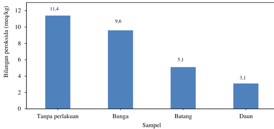
Gambar 1. Bilangan Peroksida Minyak Goreng bekas
