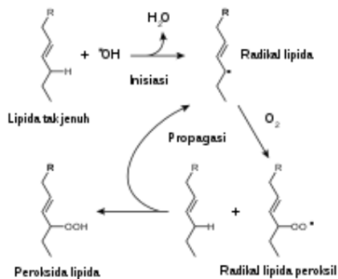
Gambar 2 Reaksi Oksidasi Minyak
