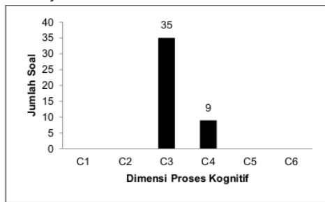
Gambar 2. Hasil Analisis Ranah Dimensi Proses Kognitif Latihan Soal pada Materi Vektor
