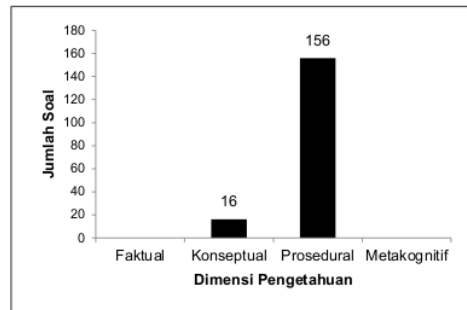
Gambar 9. Hasil Analisis Ranah Dimensi Pengetahuan Latihan Soal pada Materi Vektor, Gerak Lurus dan Gerak Parabola
