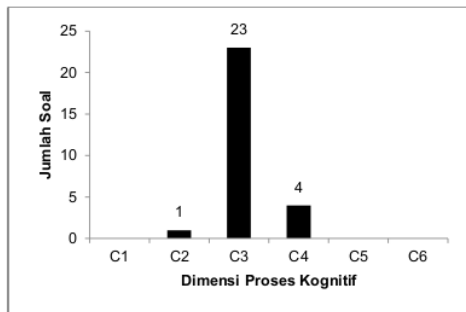
Gambar 6. Hasil Analisis Ranah Dimensi Proses Kognitif Latihan Soal pada Materi Gerak Parabola
