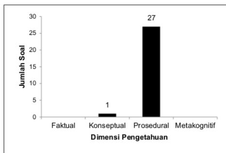
Gambar 7. Hasil Analisis Ranah Dimensi Pengetahuan Latihan Soal pada Materi Gerak Parabola
