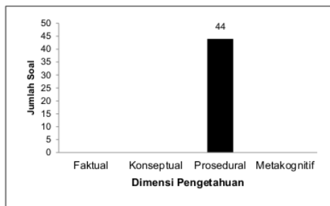
Gambar 3. Hasil Analisis Ranah Dimensi Pengetahuan Latihan Soal pada Materi Vektor
