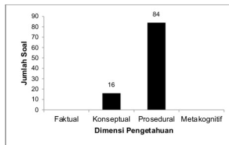
Gambar 5. Hasil Analisis Ranah Dimensi Pengetahuan Latihan Soal pada Materi Gerak Lurus
