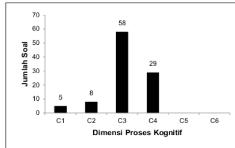
Gambar 4. Hasil Analisis Ranah Dimensi Proses Kognitif Latihan Soal pada Materi Gerak Lurus
