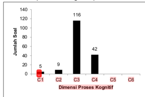
Gambar 8. Hasil Analisis Ranah Dimensi Proses Kognitif Latihan Soal pada Materi Vektor, Gerak Lurus dan Gerak Parabola
