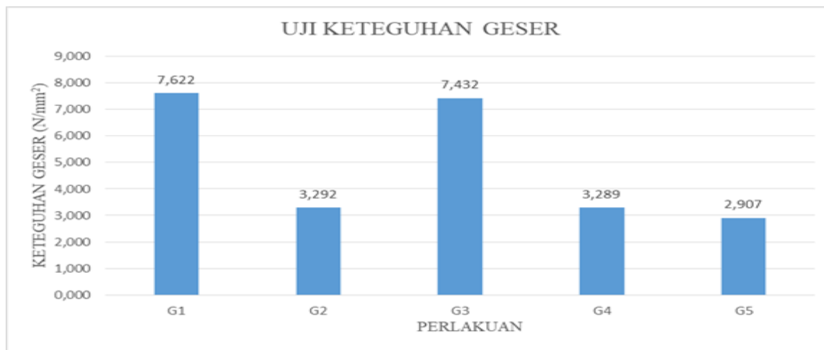
Gambar 2. Diagram Nilai Rataan Keteguhan Rekat Geser Kayu Solid dan Kayu Lamina
