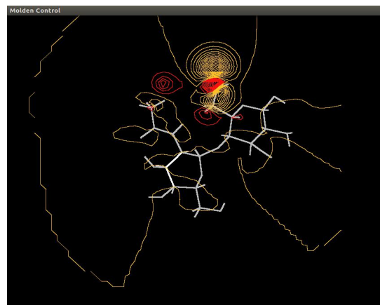
Gambar 19. Orbital Molekul kitosan + 5H^+ dilihat secara Ecluid dengan aplikasi Gmolden
