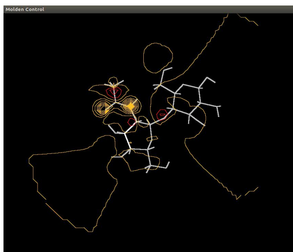
Gambar 4. Orbital Molekul kitosan dilihat secara Ecluid dengan aplikasi Gmolten
