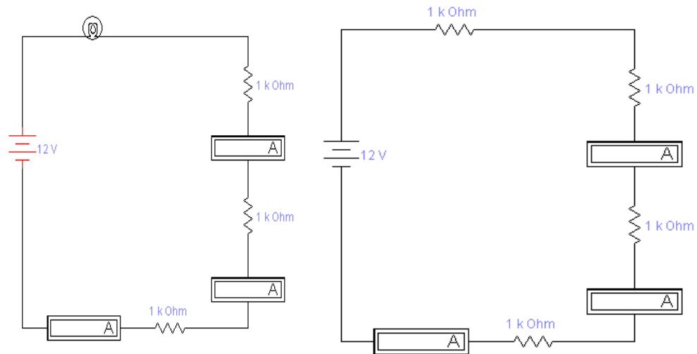
Gambar 4.2. Rangkaian Pengukuran Arus DC
