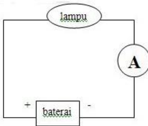
Gambar 4.1. Diagram Rangkaian DC Amperemeter
