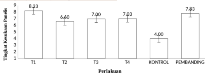
Gambar 3. Nilai Warna Kaldu Bubuk Kepala Udang Windu ( Penaeus monodon ) Dengan Berbagai Jenis Bahan Pengisi.
