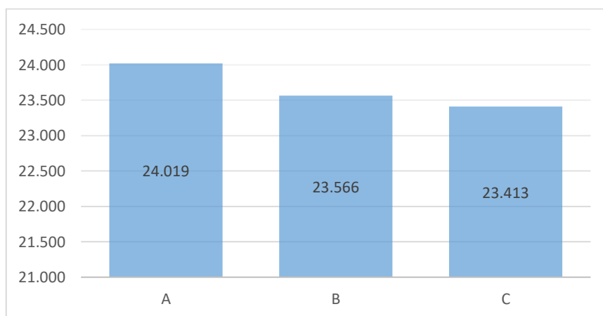
Gambar 5. Nilai rataan keteguhan tekan briket arang
