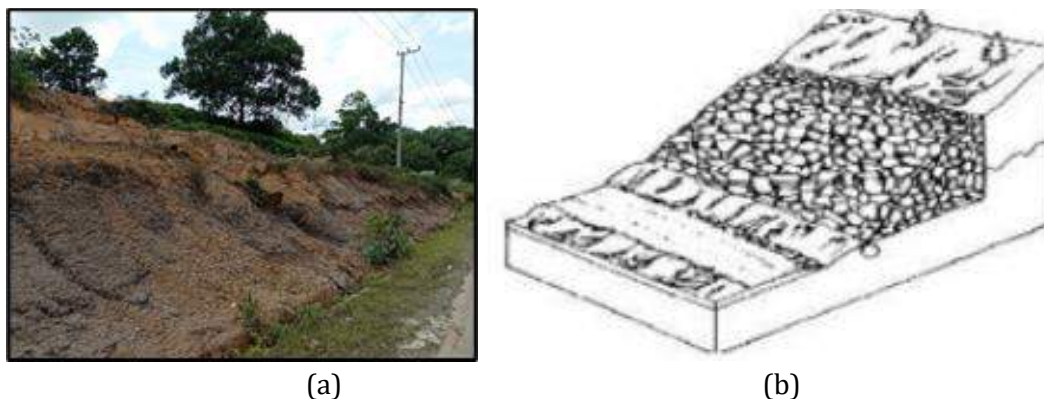
Gambar 7. (a) Lokasi Penelitian Km 19; (b). Penambatan dengan metode buttress : (Diklat Penanganan Longsor Pada Struktur Jalan)
