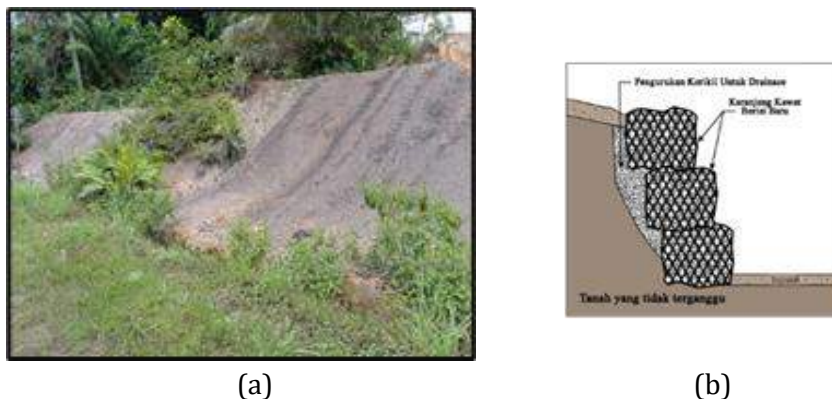
Gambar 6. (a) Lokasi Penelitian Km 18; (b). Bronjong batu (Diklat Penanganan Longsor Pada Struktur Jalan)
