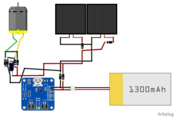
Gambar 2. Rangkaian Skematik Prototipe
