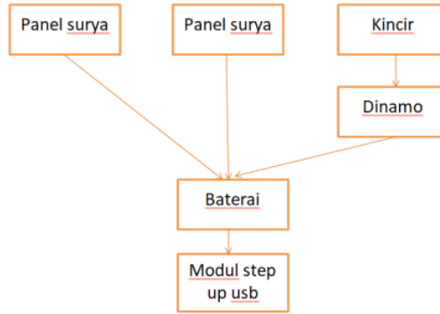
Gambar 3. Diagram Blok Alat
