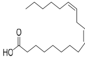
Gambar 1. Struktur kimia fraksi kloroform umbi bawang tiwai pada pengujian dengan GC-MS (9,12-Octadecadienoic Acid (C 18 H 31 O 2 ))
