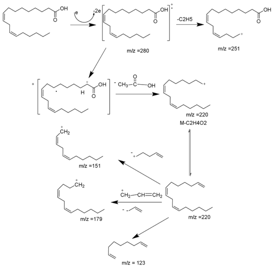
Gambar 2. Pola Fragmentasi senyawa 9,12-Octadecadienoic Acid (C 18 H 31 O 2 )
