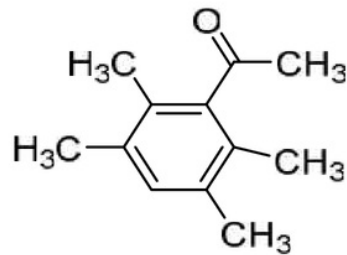
Gambar 3. Struktur kimia fraksi kloroform umbi bawang tiwai pada pengujian dengan GC-MS (1-(2,3,5,6-Tetramethylphenyl) Ethanone (C 12 H 16 O))
