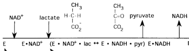
Gambar 1. Mekanisme reaksi enzimatik DHL
