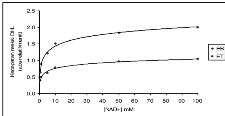
Gambar 3. Pengaruh variasi konsentrasi NAD + dengan menjaga konsentrasi L-laktat tetap 0,1 M terhadap kecepatan reaksi enzim DHL bebas (EB) dan enzim DHL terenkapsulasi (ET)
