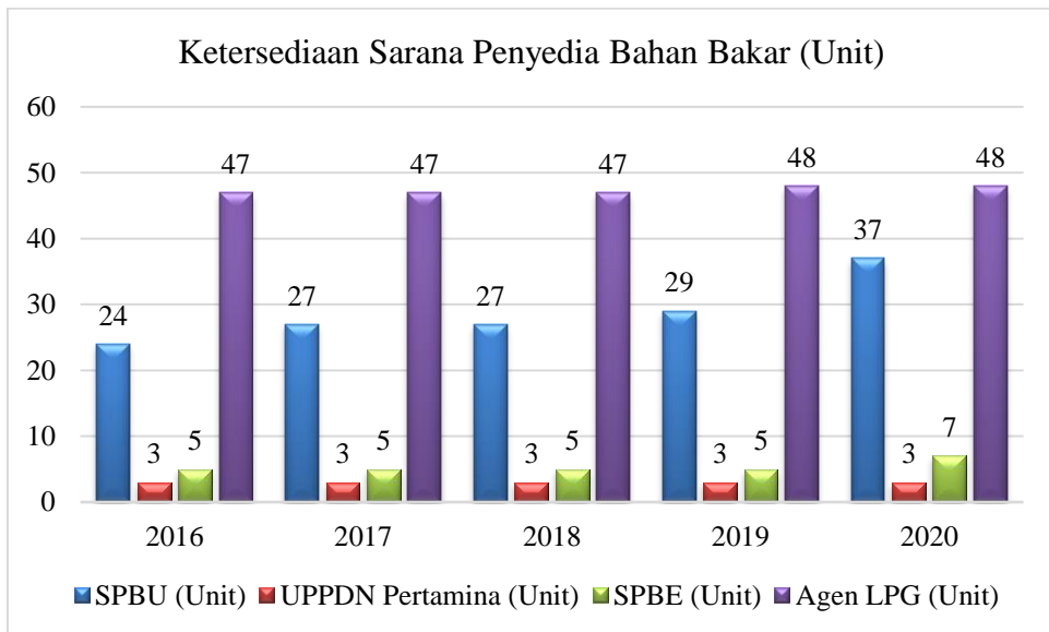
Gambar 56. Grafik Ketersediaan Sarana Penyedia Bahan Bakar (Unit)
