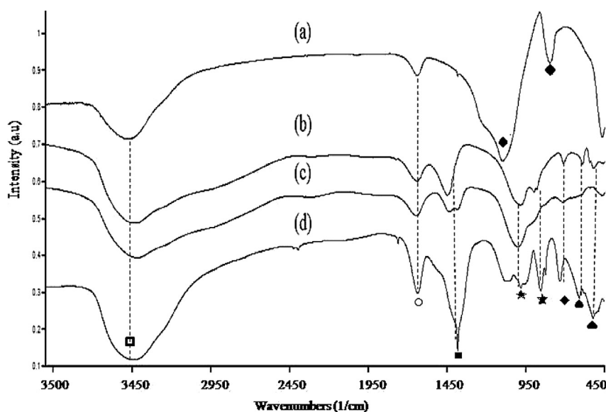
Fig. 1. FT-IR spectra of (a) RHS, (b) \text{K}_2\text{SiO}_3 , (c) \text{Na}_2\text{SiO}_3 , (d) \text{Li}_2\text{SiO}_3 ; \blacktriangle : \text{M}^+\text{--O} ; \blacklozenge : \text{O--Si--O} ; \star : deformation ( \text{Si--O--Si--(M--O)} ); \blacksquare : \text{Si--O--Si} stretching; \circ : \text{O--H} vibration from water molecules; \square : \text{O--H} bending and stretching (after calcined at 500^\circ\text{C} ).
